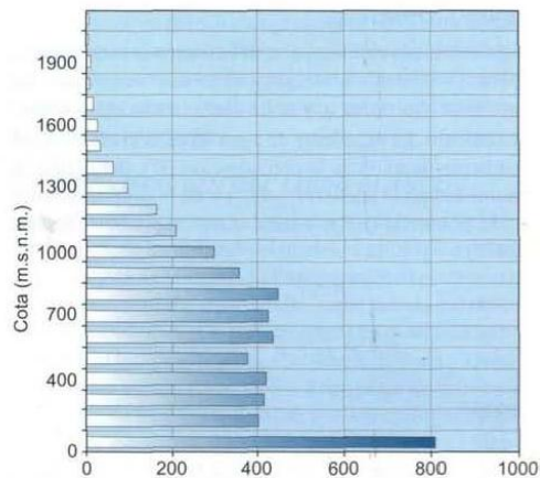
Figura 4. Distribución de las estaciones meteorológicas según su altitud
