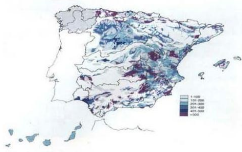
Figura 18. Mapa de capacidad de infiltración máxima (mm)
