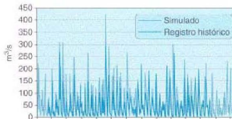
Figura 21. Series mensuales simuladas e históricas del río Miño en Lugo (periodo 1940 ... 1995)
