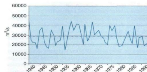
Figura 39. Recarga por infiltración de lluvia ( hm^3/año ) en la Península (periodo 1940/41 a 1995/96)
