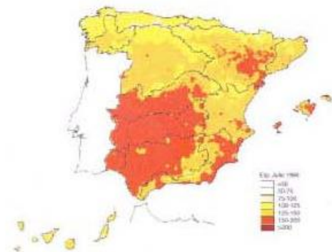
Figura 11. Cálculo de la ETP (mm) según Thornthwaite (julio 1990)
