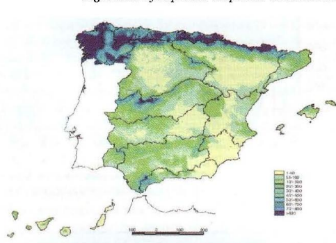
Figura 31. Mapa de escorrentía total media anual en mm (periodo 1940-1995)
