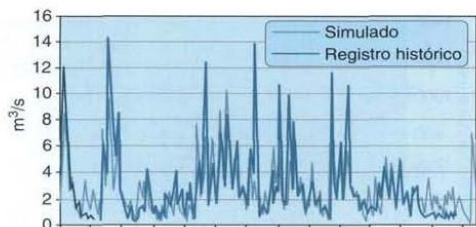
Figura 23. Series mensuales simuladas e históricas del río Guadalquivir en La Cubeta (periodo 1940 – 1995)
